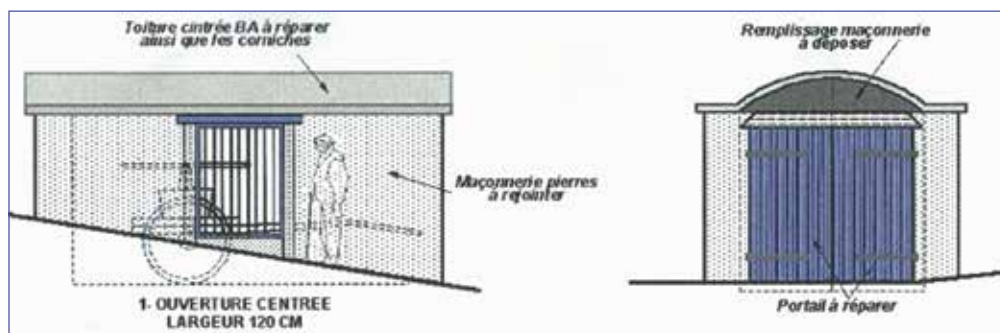
Projet du local de la pompe à incendie.
